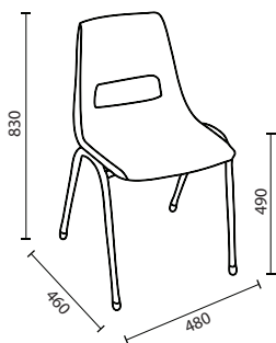
Shell Sled SS01
